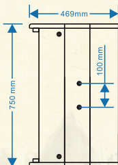
侧视图
